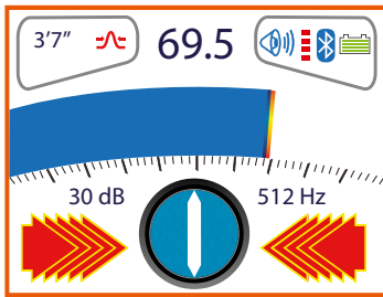
vLocPro2
